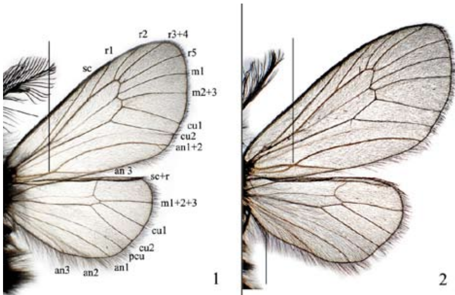
Fig. 1-2. Nervature ala anteriore: connessione fra an1+2 e an3 .
